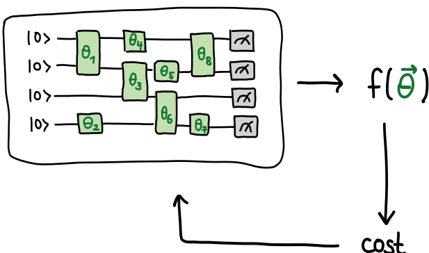
Visualisierung eines Quanten-Variationsalgorithmen-Schaltkreises.
